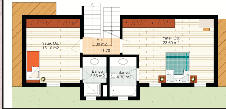
-1.70 Kotu Kat Planı
